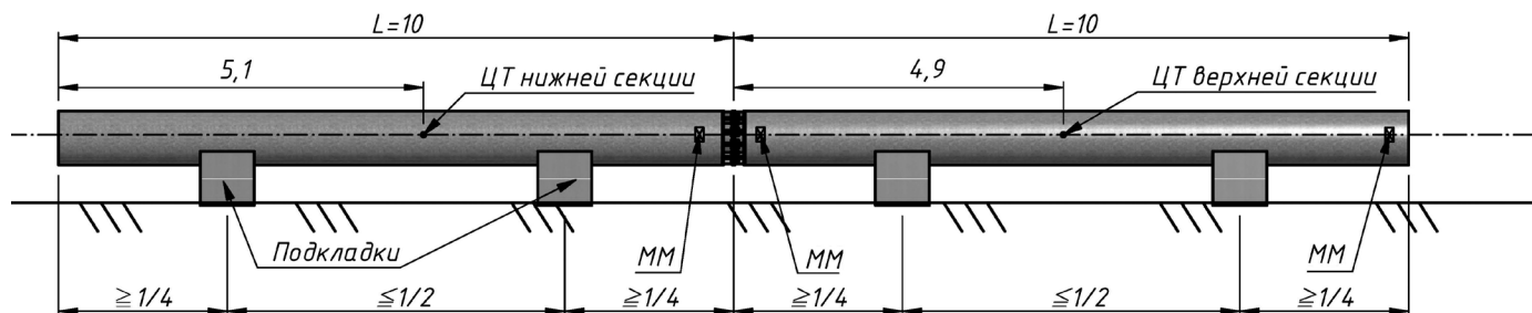
Схема сборки секционированной стойки СЦ20 (Ф800)
