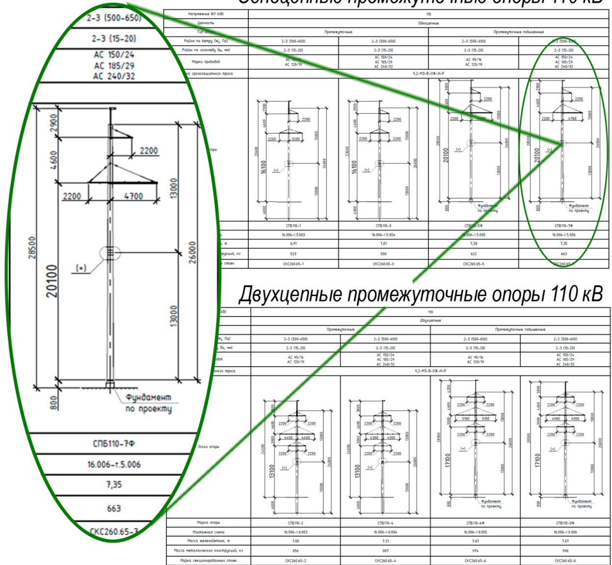
Рис. 2. Обзорный лист промежуточных опор
