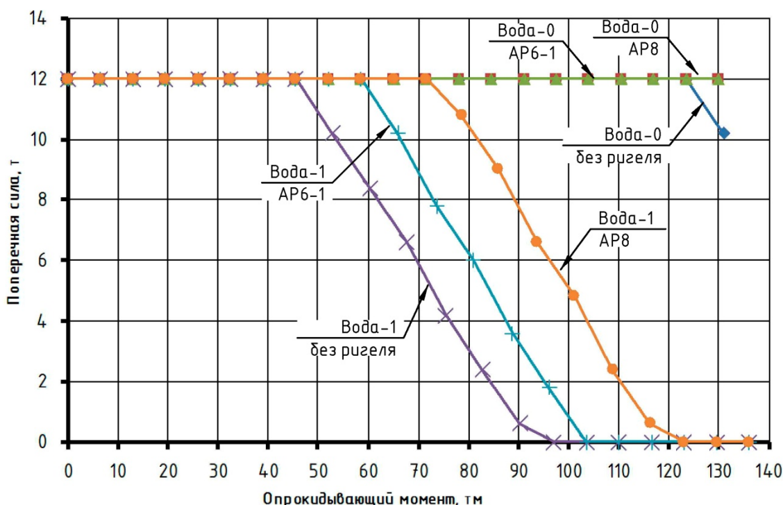
Рис. 5. График несущей способности по грунту для фундамента под промежуточную опору длиной 5 м
