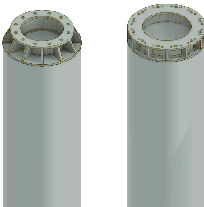
Рис.4. Фундаментные секций для установки промежуточных и анкерно-угловых железобетонных опор
